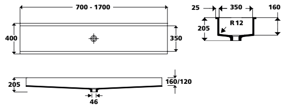
Unterbauwaschrinne 350
