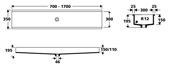
Unterbauwaschrinne 300
