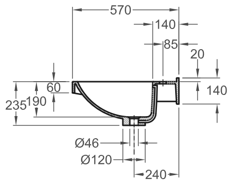
VARICOR Werset Waschtisch-Schnitt 08.03.2005/Re
