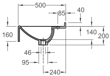
VARICOR Tangent Waschtisch-Schnitt 23.02.2005/Re
