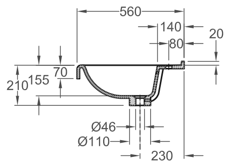
VARICOR Preciosa Pro Waschtisch-Schnitt 22.04.2004/Re
