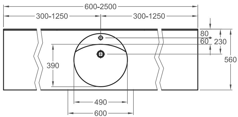
VARICOR Preciosa Pro Einzelwaschtisch Becken mittig, rechts oder links 19.10.2011/Re-Th
