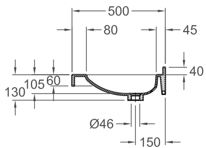
Florac Waschtisch gerundet-Schnitt 19.10.2011/Th
