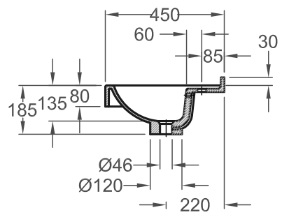
VARICOR AKZENT Waschtisch-Schnitt 17.10.2011/Re-Th
