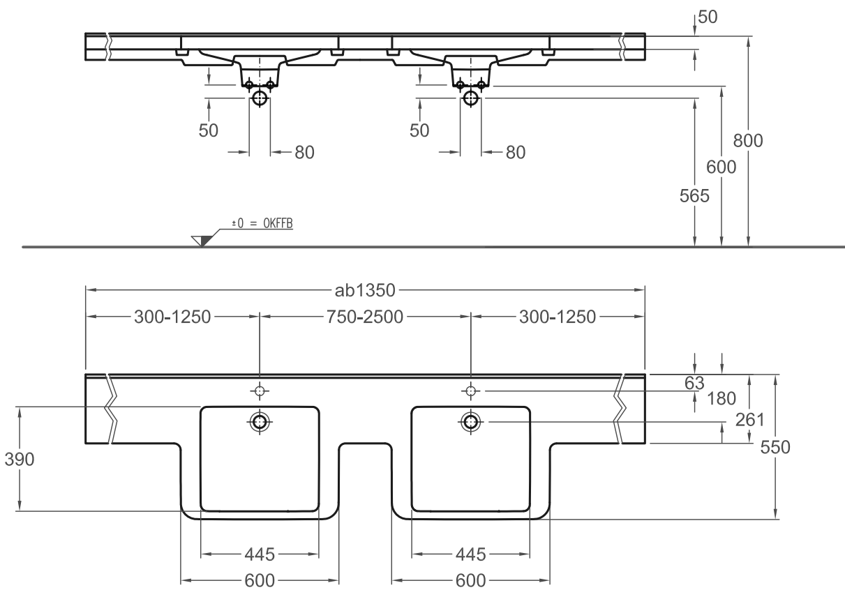
Dejuna Pro Doppelwaschtisch mit seitlichen Ablageflächen / a 19.10.2011/Th
